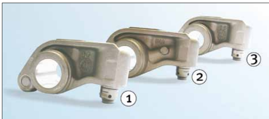
Slika 1: Pregled tri razna KIT-a poluge ventila
