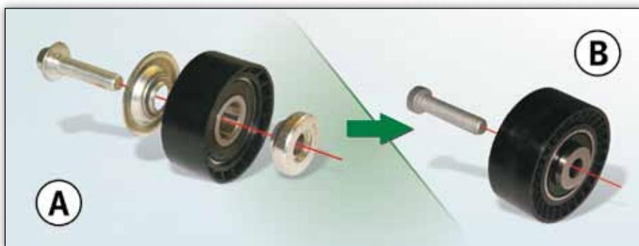
Slika 1: Klizač sa kat. Br. 532 0433 10, dosadašnja izvedba (A) i nova izvedba (B)
