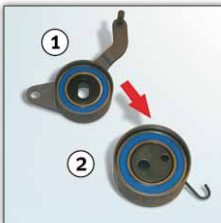
Slika 1: Dosadašnja natezna rolica Kat. Br. 531 0166 20 (1) je zamjenjena sa nateznom rolicom Kat. Br. 531 0819 10 (2)
