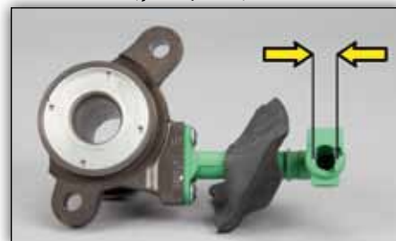
Slika 4: LuK CSC 510 0137 10 hidraulični priključak Ø 12,2 mm/Ø 13,3 mm, Ø 11,7 mm/Ø 12,2 mm
