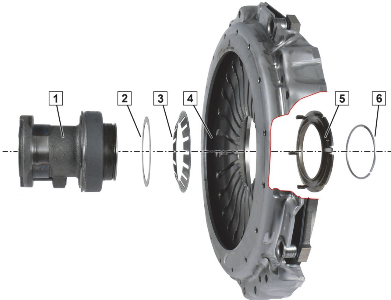
Sl. 1: isključivač s čvrstim spojem, redoslijed montaže i orijentacija dijelova
